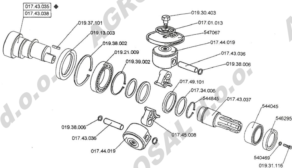
ČRPALKA BM 105/20
