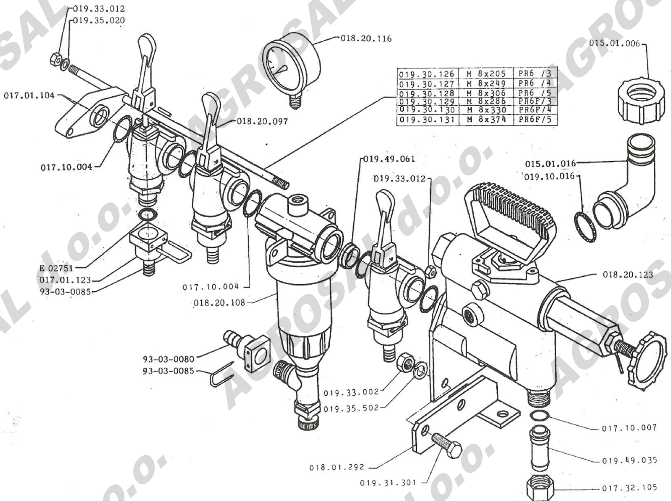
PRETOČNI REGULATOR PR-6
