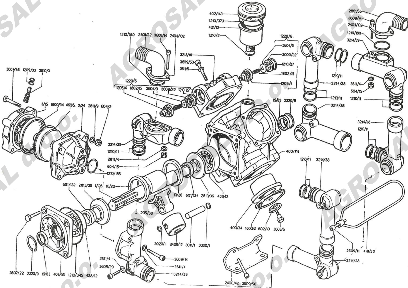
ČRPALKA BP 151
