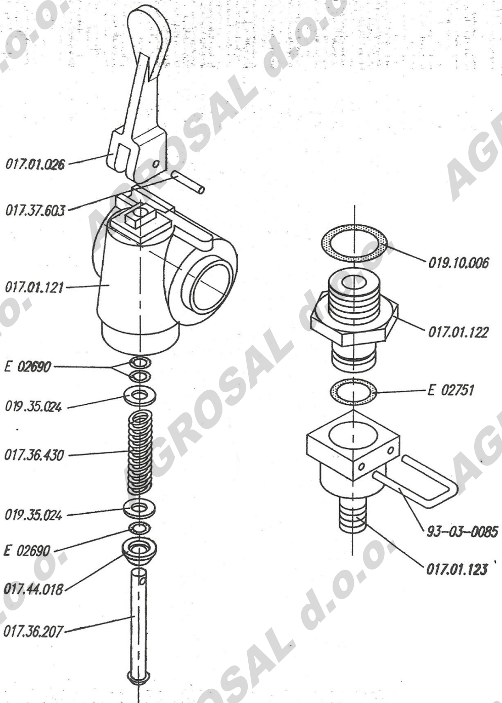
VENTIL RAZVODNI PR-1
