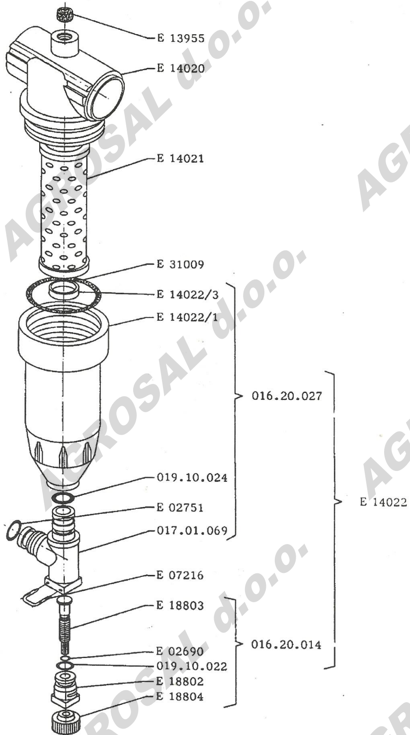
FILTER SAMOČISTILNI NIZKOTLAČNI
