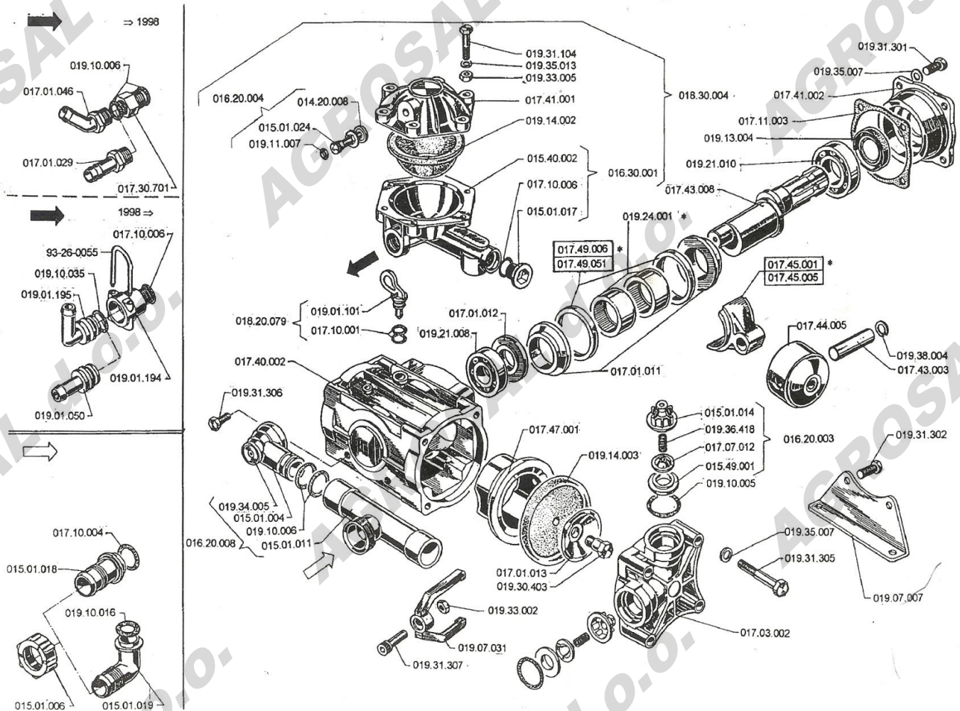
ČRPALKA BM 65/20 STD
