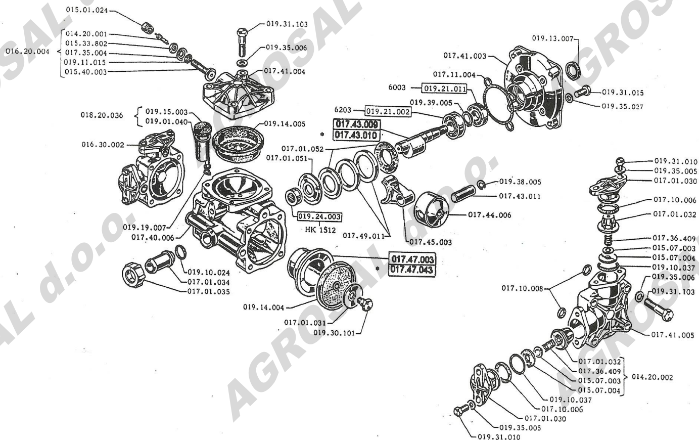
ČRPALKA BM 20/15
