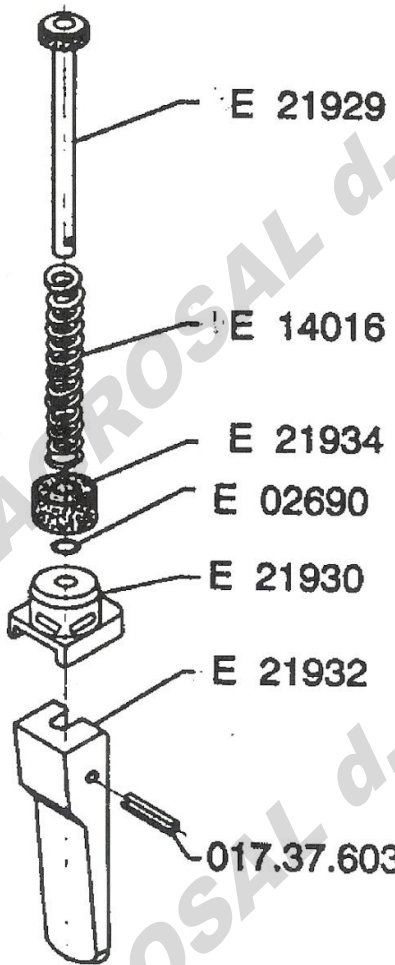
VENTIL RAZVODNI PR-3
