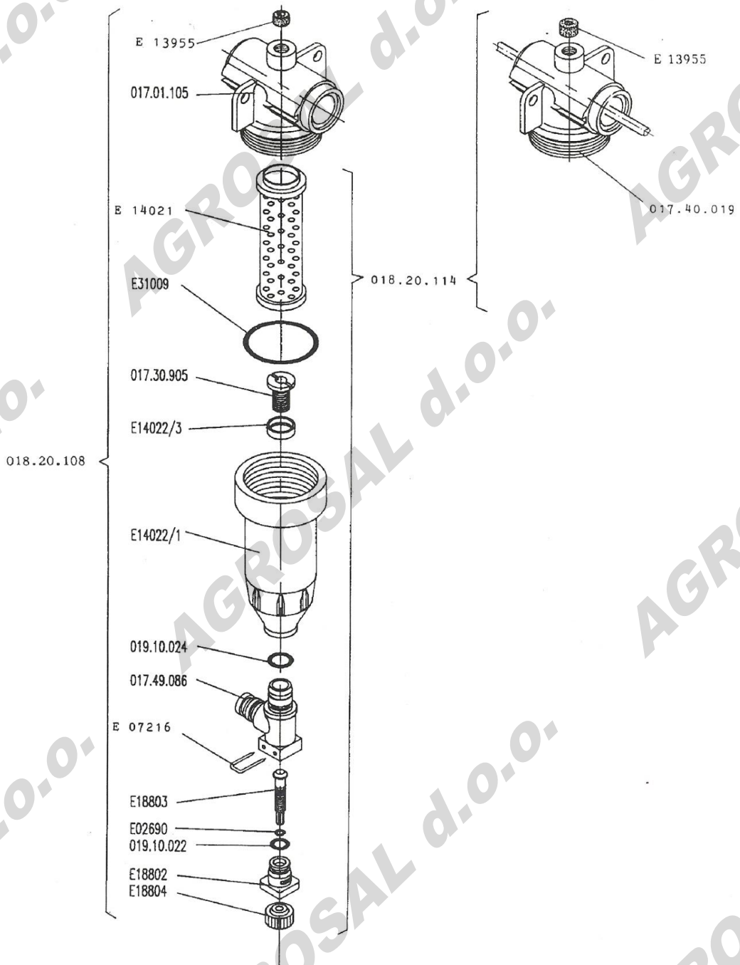
FILTER SAMOČISTILNI VISOKOTLAČNI
