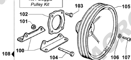
Varianti / Version Albero Passante 6 Fori Cilindrico Ø25 6 Holes Throughshaft Ø25 Cylindric
