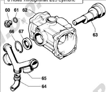
Varianti / Version Albero Passante 6 Fori Cilindrico Ø25 6 Holes Throughshaft Ø25 Cylindric
