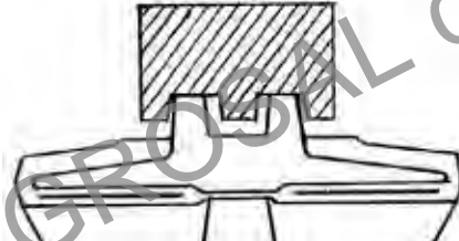
LOW OUTER DOUBLE FLANGE TRACK ROLLER RULLO DOPPIO BORDO GUIDA ESTERNA
