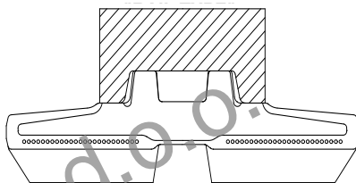
"RAIL TYPE" OUTER DOUBLE FLANGE TRACK ROLLER RULLO DOPPIO BORDO GUIDA ESTERNA ALTA "RAIL"
