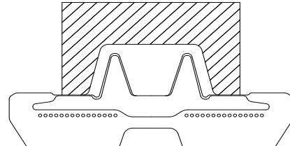
LOW OUTER DOUBLE FLANGE TRACK ROLLER RULLO DOPPIO BORDO GUIDA ESTERNA
