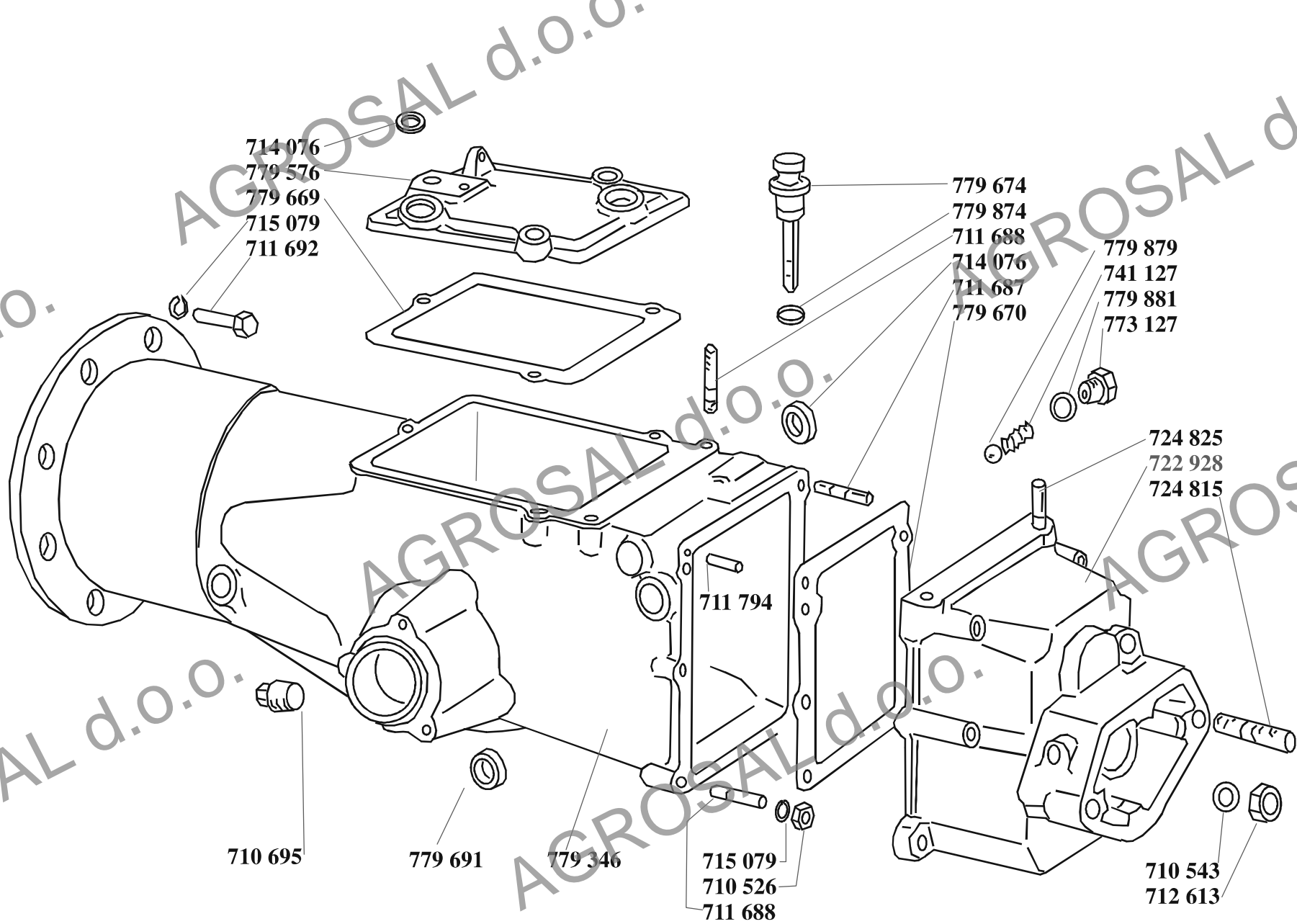
OHIŠJE Z DIFERENCIALOM
